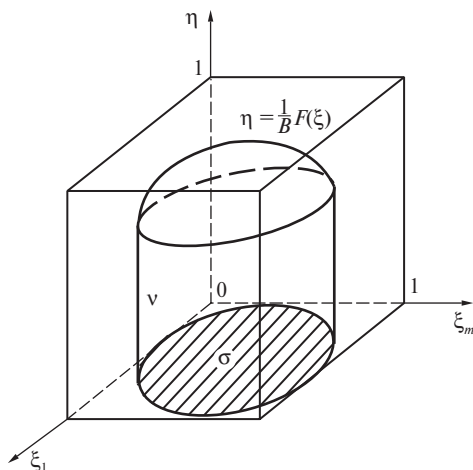
Рис. 5.5. Цилиндрои пространства O\xi_1\xi_2\dots\xi_m\eta , построенный на области \sigma и ограниченный снизу гиперплоскостью \eta = 0
